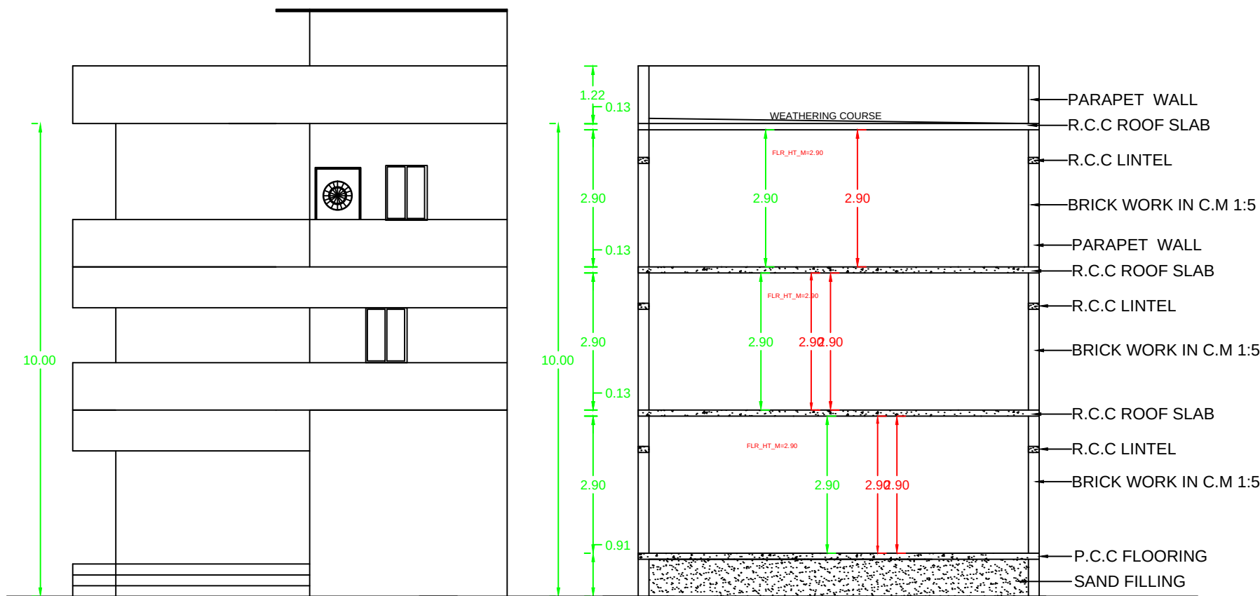
ELEVATION
