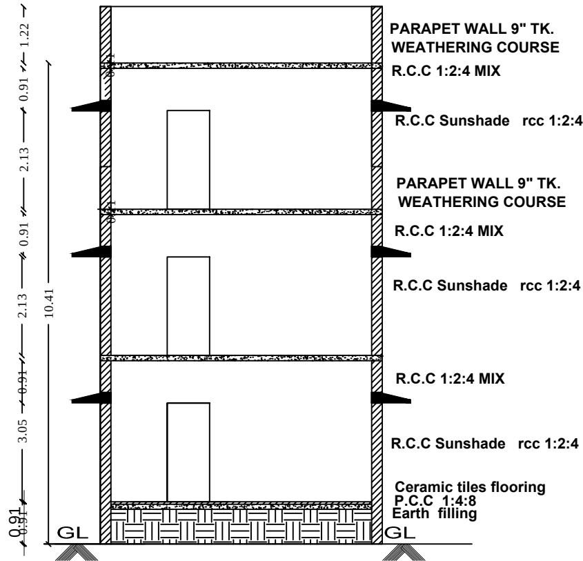
SECTION A-A'
