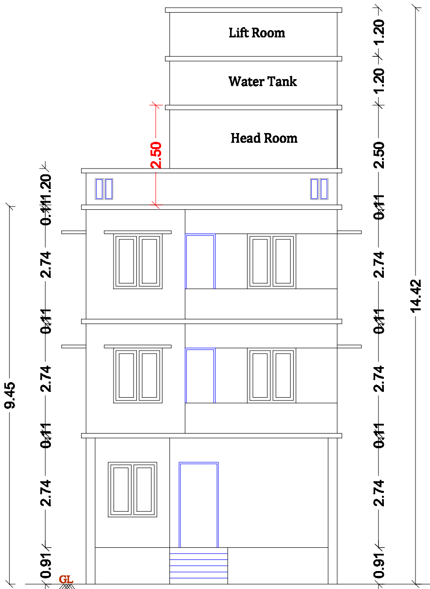
ELEVATION
