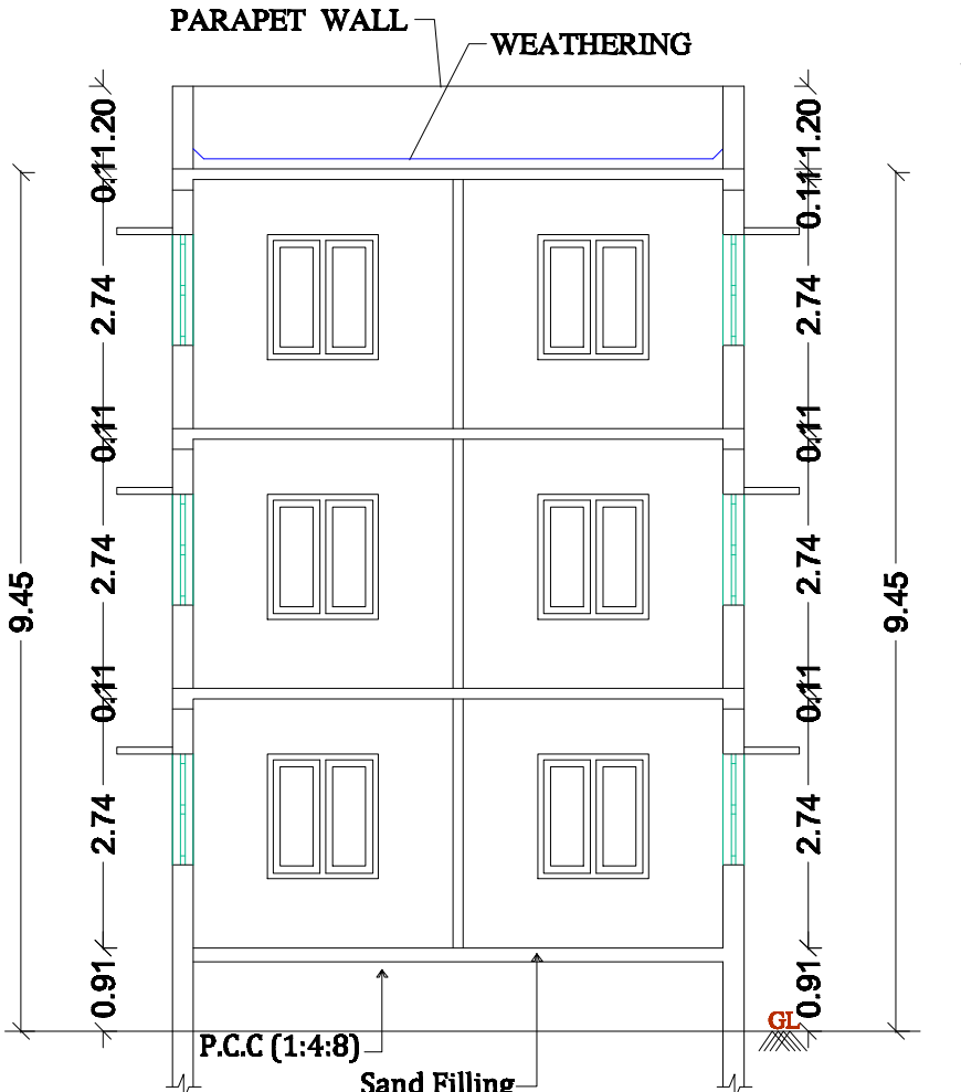
SECTION A-A
