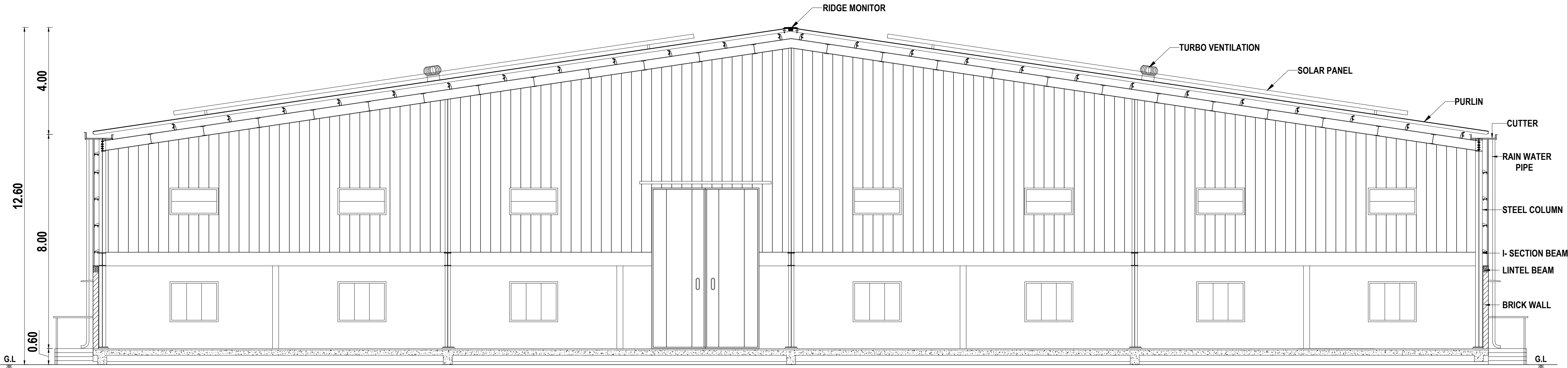
CROSS SECTION - A. A'
