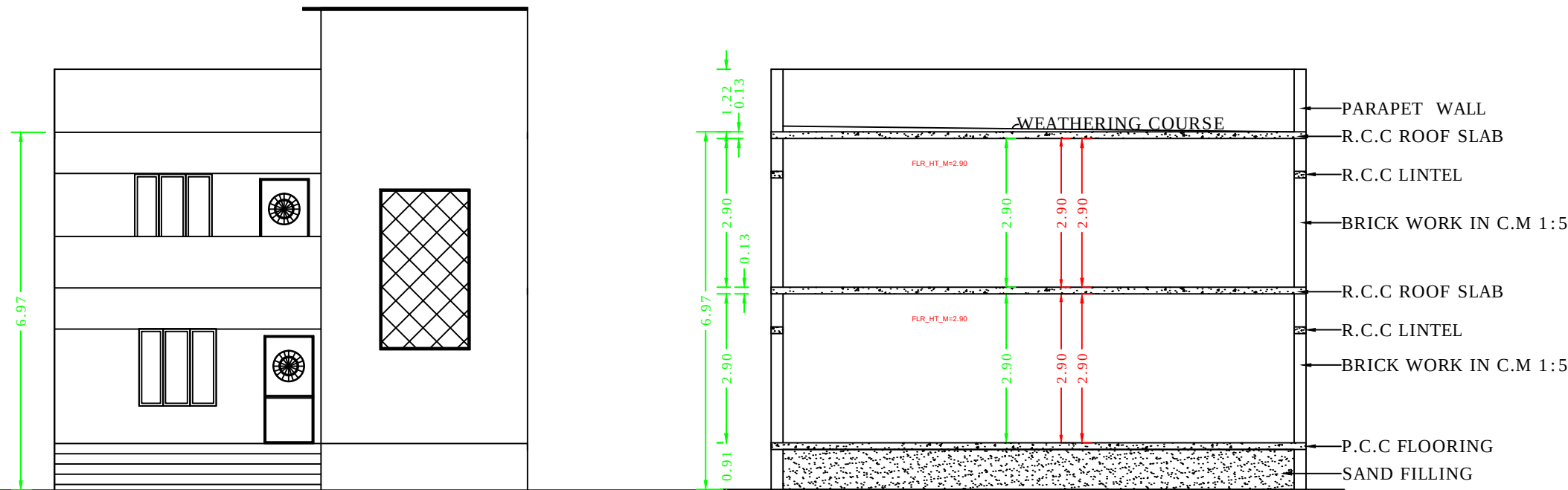
ELEVATION
