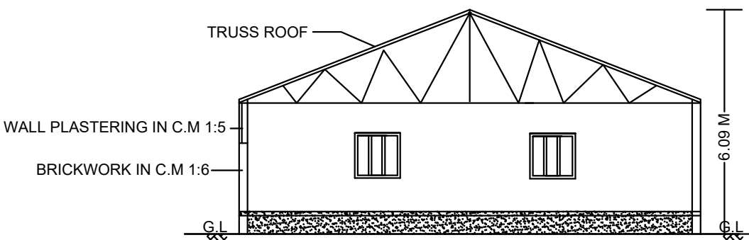
SECTION S.P
