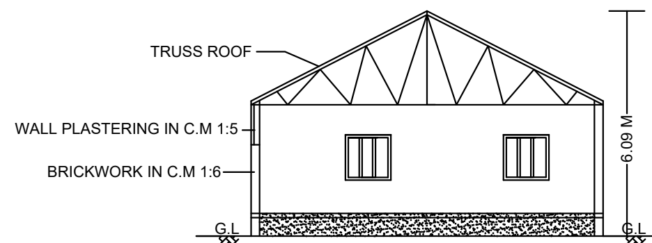
SECTION S.P
