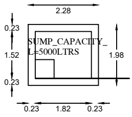
SUMP
