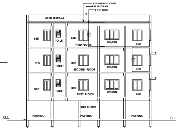
SECTION A-B
