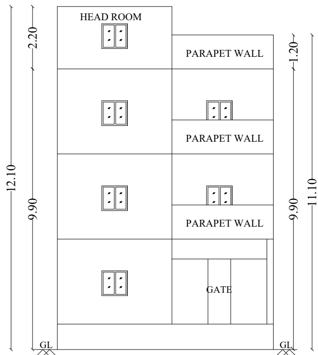
ELEVATION
