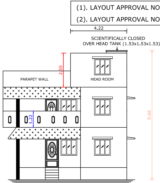
ELEVATION
