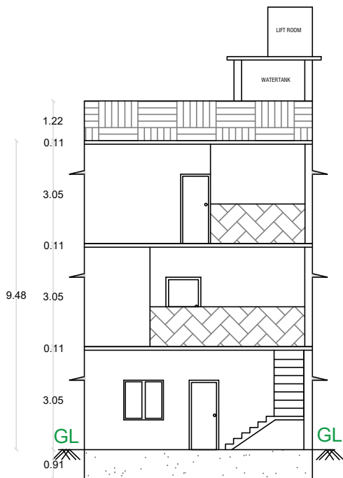
ELEVATION
