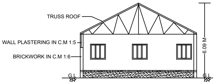
SECTION S.P
