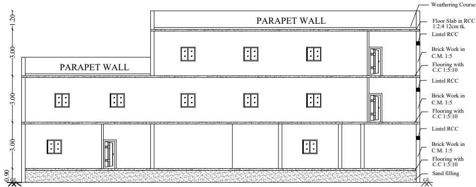
SECTION A-A
