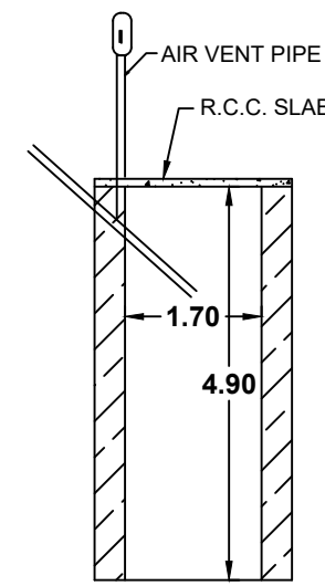
SOAK PIT
