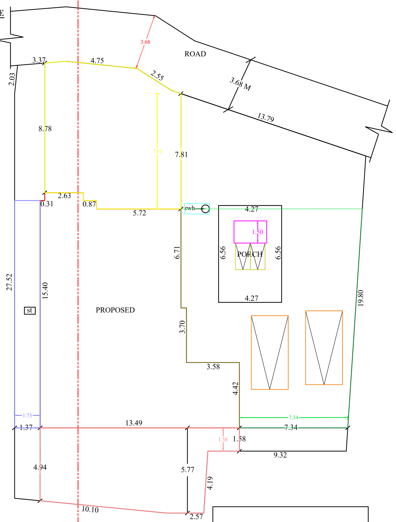
SCALE 1:100 SITE PLAN
