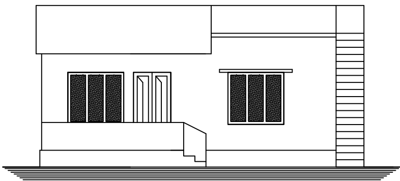
ELEVATION
