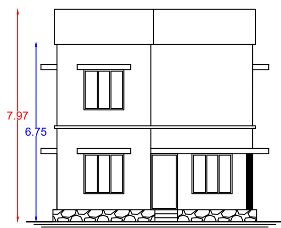
ELEVATION
