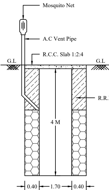
SOAK PIT
