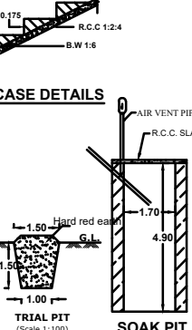
SOAK PIT
