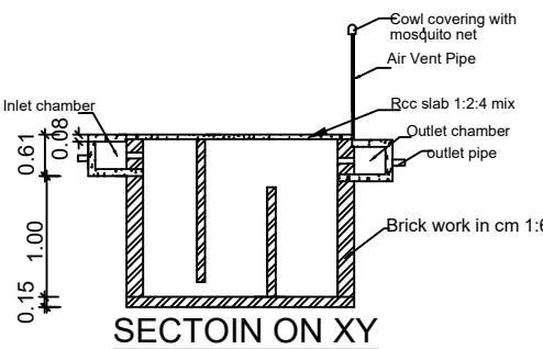
SECTOIN ON XY
