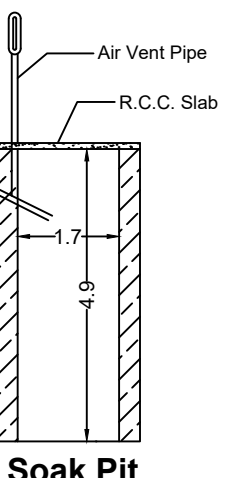
Soak Pit
