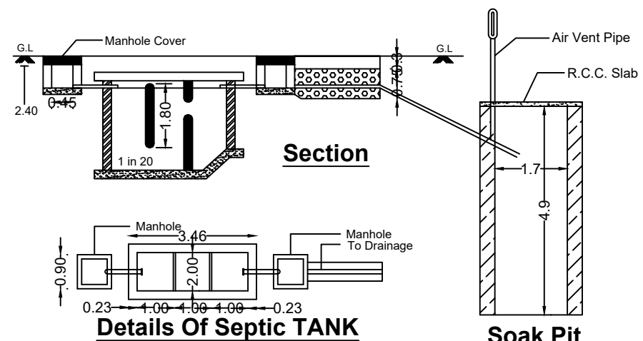
Soak Pit
