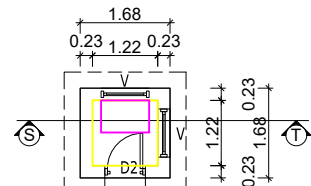
TOILET PLAN
