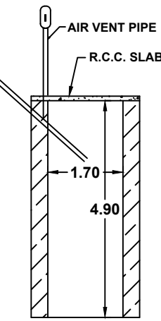
SOAK PIT
