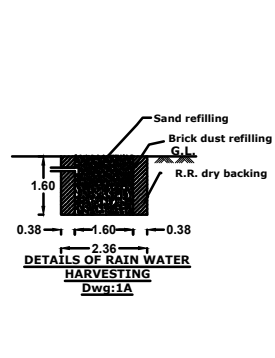
SOAK PIT
