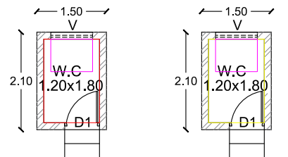
GENTS TOILET PLAN
