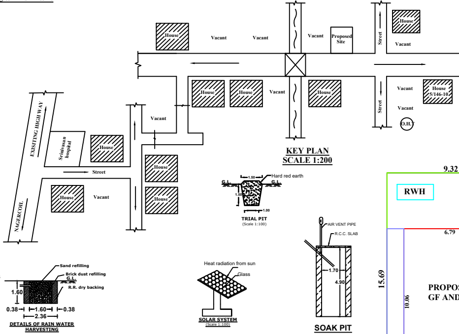
SOAK PIT
