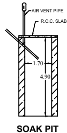
SOAK PIT
