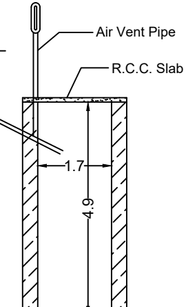
Soak Pit
