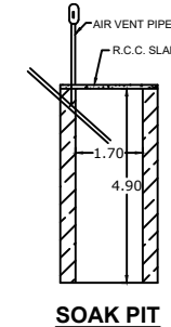
SOAK PIT
