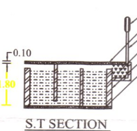
S.T SECTION
