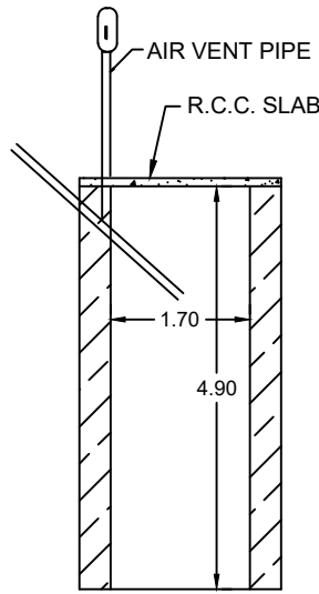
SOAK PIT
