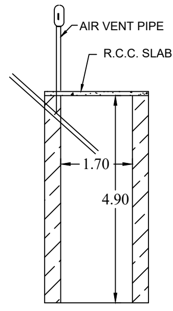
SOAK PIT
