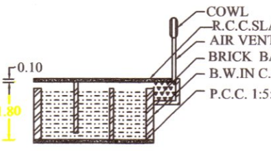
S.T. SECTION
