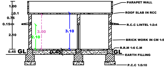
SECTION -AB
