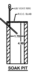
SOAK PIT
