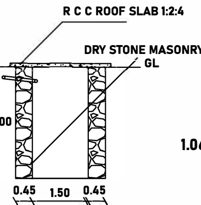
SOAK PIT
