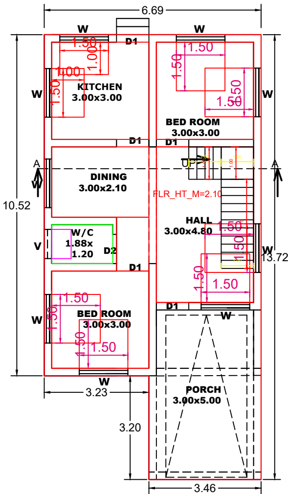
G. F. PLAN
