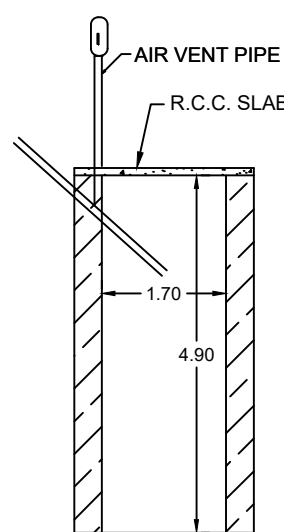
SOAK PIT
