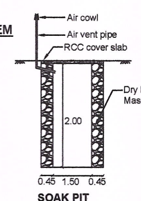
SOAK PIT
