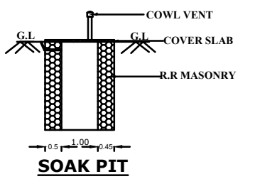
SOAK PIT
