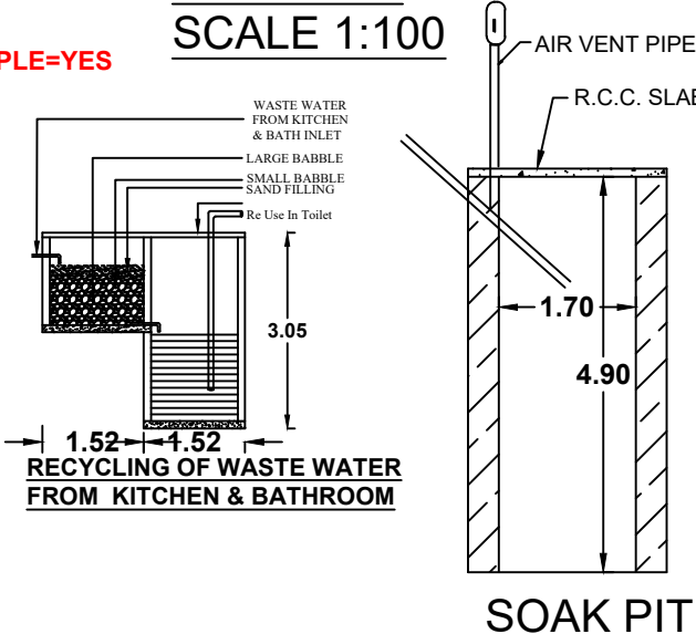
SOAK PIT
