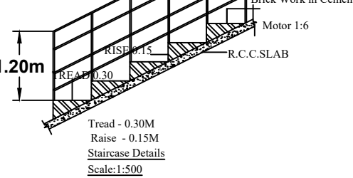
Staircase Details Scale: 1:500
