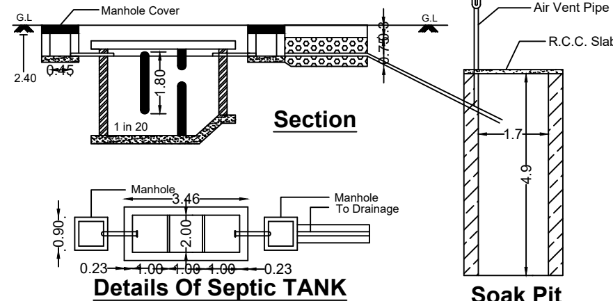
Soak Pit
