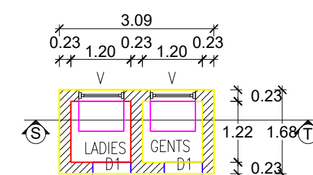
TOILET PLAN
