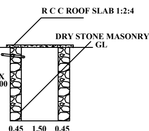
SOAK PIT
