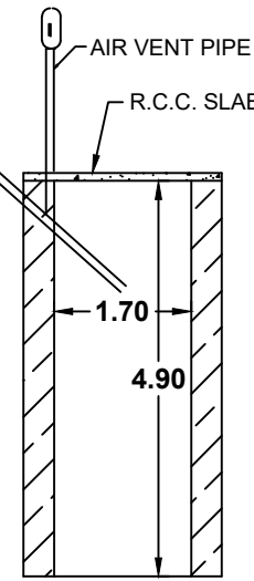
SOAK PIT
