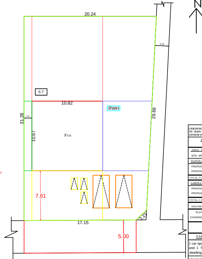
SCALE 1:100 SITE PLAN
