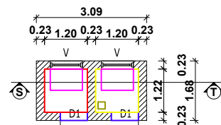
TOILET PLAN
