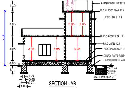
SECTION - AB
